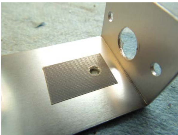
② 絶縁シートを貼ります
