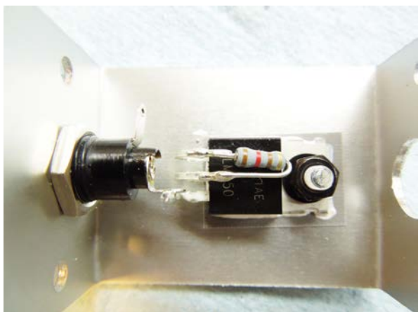
⑥ 120Ω、入力コネクタ+極 半田付け
