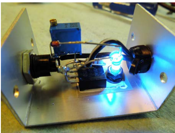
⑫ 出力に 1.5kΩを直列接続した LED を接続
