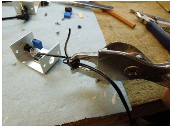
⑨ 出力ケーブル・ブッシング挿入
