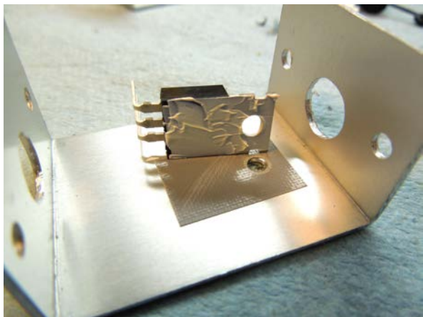
③ 放熱シリコン塗布(キットに含まず)
