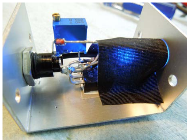
⑬ 黒色アセテートテープで覆う
