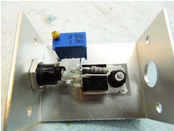
⑧ VR 位置 整形
