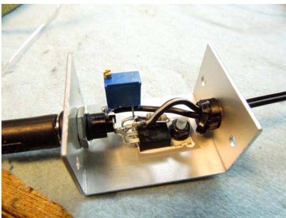
⑩ 出力ケーブル 半田付け
